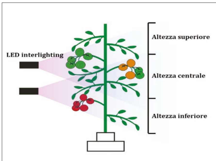
Schema grafico del posizionamento delle lampade Led interlighting
